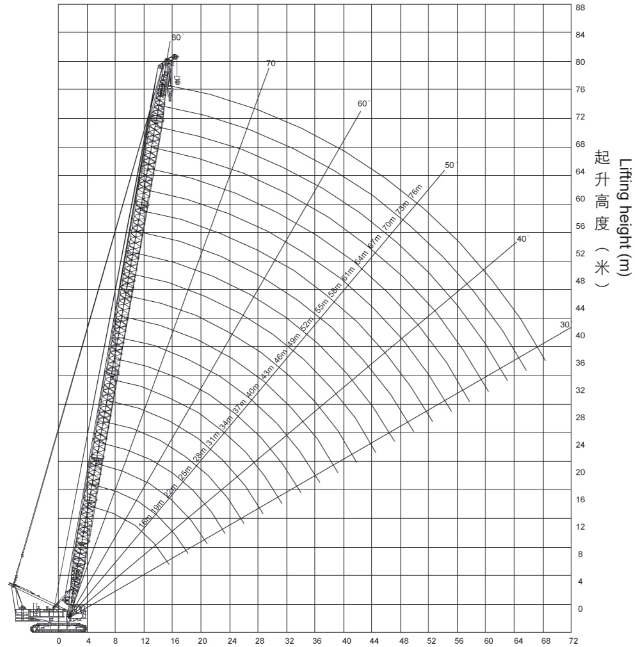
工作幅度 (米) Working radius (m)
